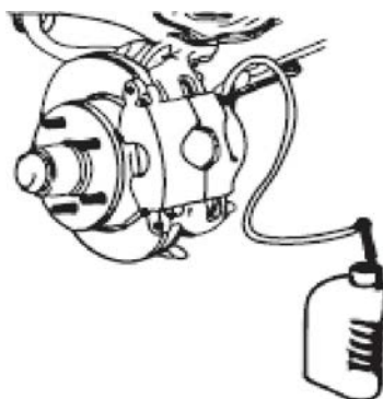
Рис. 5 Прокачка гидравлической тормозной системы
